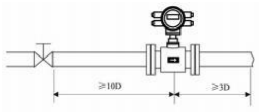
图 10 阀门位于传感器上游的安装
