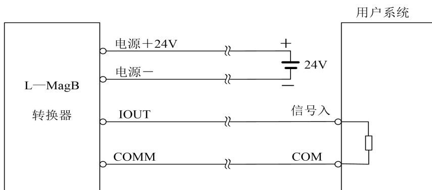
图 7.6.3 (c) L-magB 四线制接法 (供电和电流输出隔离方式)
