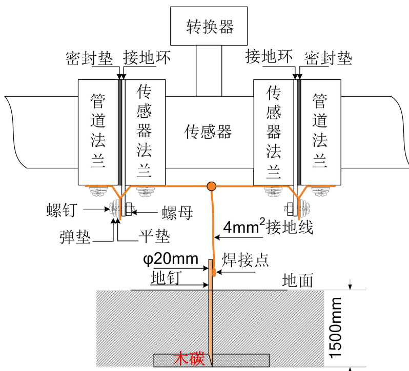
图 7.4.4 转换器接地示意图
