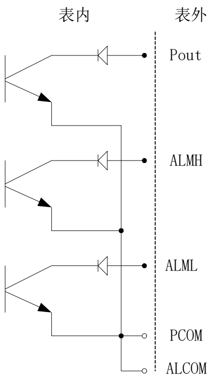
图 7.3.3 (e) 表内 OC 门连接方式
